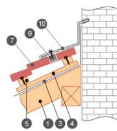
Устройство вентилируемого конька
