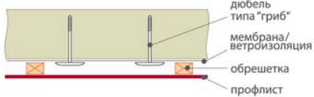
Неутепленный фасад
