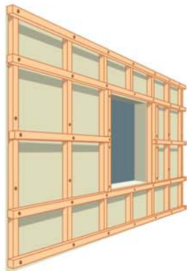
Деревянная обрешетка
