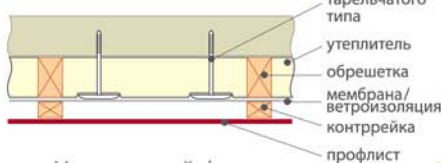
Утепленный фасад
